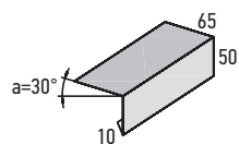
Фартук S1 карнизный развертка 12,5 см, длина 2 м
