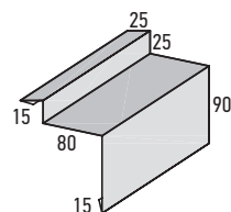
Фартук S20 пристенного аэратора в штрабу развертка 25 см, длина 2 м
