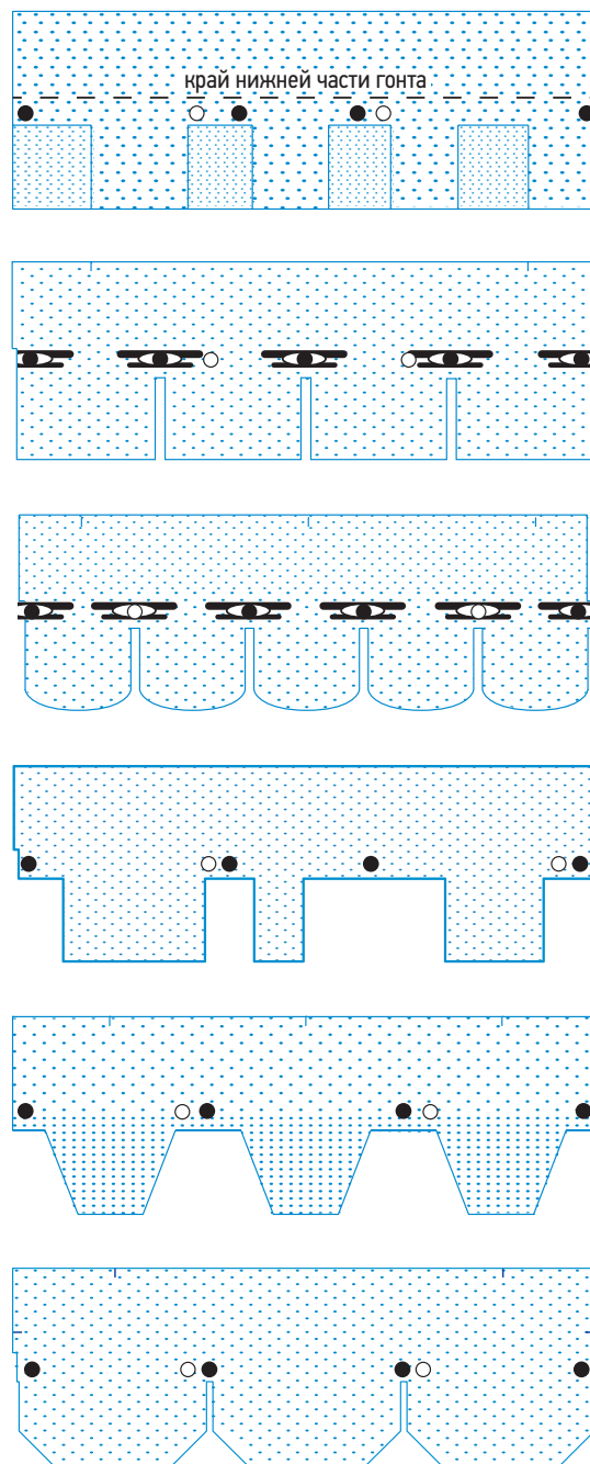
Уклон кровли более 60°
