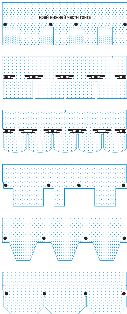
Уклон кровли менее 60°
