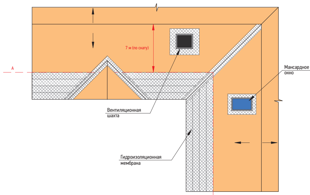
Рис. 2.22. Частичный с дополнительными рядами гидроизоляции по карнизу крыши
